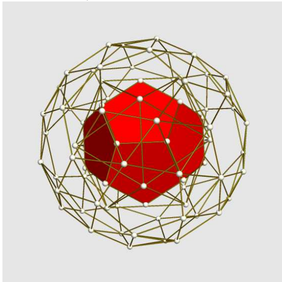
Dieser 95-Kugler ist ein gedehntes Snub Dodekaeder und hat den Radius 2.27
