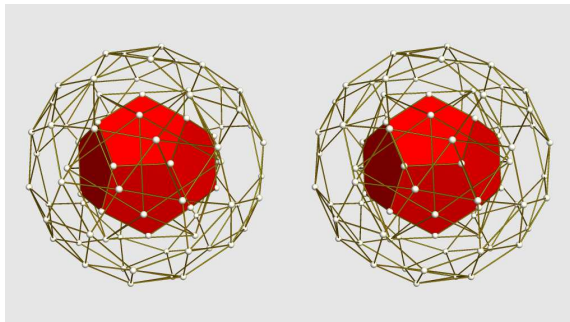
Dieser 95-Kugler ist ein gedehntes Snub Dodekaeder und hat den Radius 2.27
