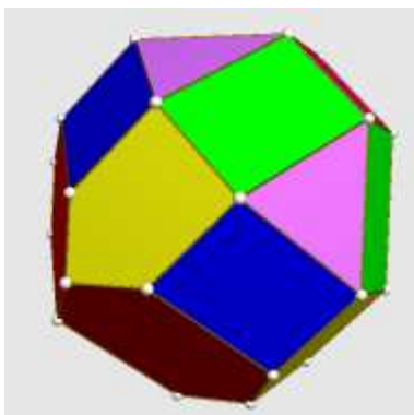
Dieser 100-Kugler hat den Radius 2.474.
